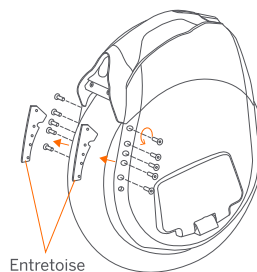
Entretoise
